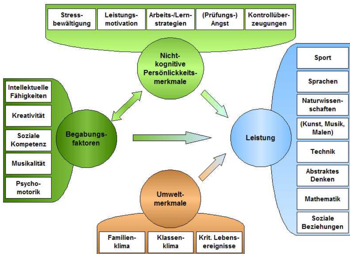
Münchner Hochbegabungsmodell
